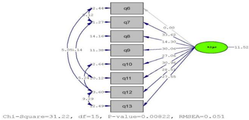
شکل ۳. مقادیر t تحلیل عاملی تأییدی مرتبه اول عامل «موده (محبت و ابراز محبت)»
