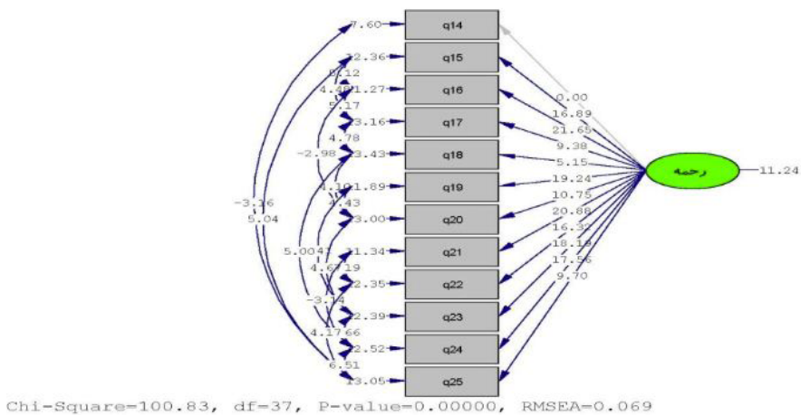
شکل ۴. مقادیر t تحلیل عاملی تأییدی مرتبه اول عامل «رحمه»
