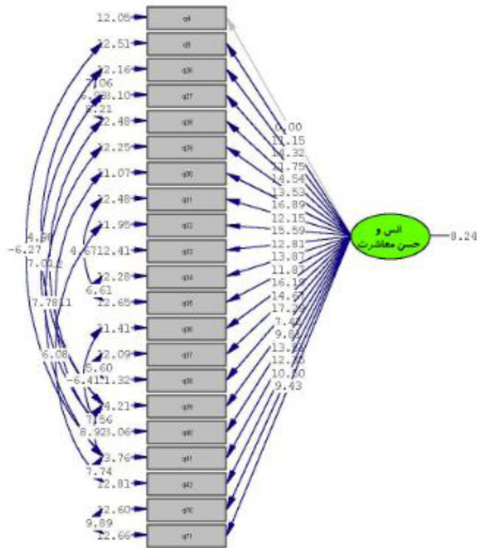
شکل ۲. مقادیر t تحلیل عاملی تأییدی مرتبه اول عامل «انس و حسن معاشرت»
