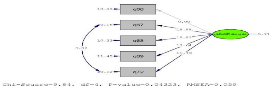
شکل ۸. مقادیر t تحلیل عاملی تأییدی مرتبه اول عامل «مدیریت اقتصادی»
