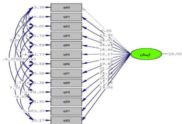
شکل ۱۰. مقادیر t تحلیل عاملی تأییدی مرتبه اول عامل «ایمان»
